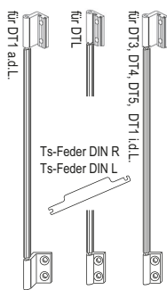
Art.Nr. B460 Schließhilfe für Drehtür Beschlagsatz 4-teilig
