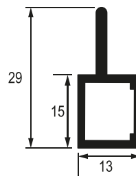
Art.Nr. A1103 Einbaurahmenprofil für Schiebetüre
