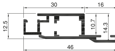
Art.Nr. A1220 Drehrahmenprofil mit Falz
