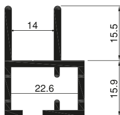
Art.Nr. A1330 Einbaurahmenprofil für Schiebetüre
