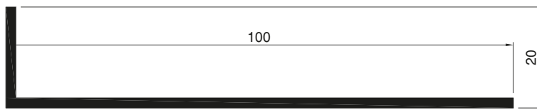
Art.Nr. A8120 L - Winkelprofil 100x20x2
