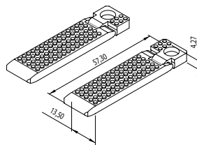
Art.Nr. B612 Klappgriff
