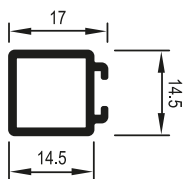
Art.Nr. A1490 Einbaurahmenprofil für Duplextüren
