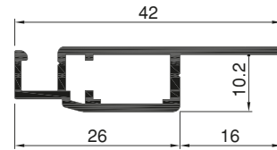
Art.Nr. A1014 Spannrahmenprofil mit Falz 16 mm
