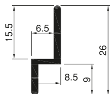
Art.Nr. A1350 Z - Profil Führungsschiene für Schiebetüre
