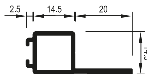
Art.Nr. A1470 Einbaurahmenprofil mit Falz für Duplextür
