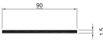
Art.Nr. A1290 Trittschutzblech
