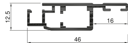
Art.Nr. A1230 Drehrahmenprofil mit Falz innen
