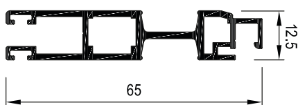
Art.Nr. A1320 Schieberahmen
