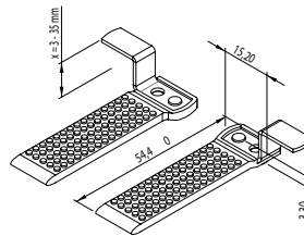
Art.Nr. B230 Mittelarretierung
