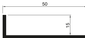
Art.Nr. A8515 L - Winkelprofil 50x15x2
