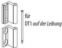
Art.Nr. B430 Scharniersatz, für Türe ohne Falz, Beschlagsatz 3-teilig
