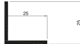
Art.Nr. A8225 L - Winkelprofil 25x25x2
