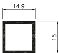
Art.Nr. A1515 RR - Hohlpr.- Einbaur. 15x15x1.2
