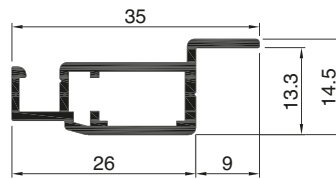
Art.Nr. A1019 Spannrahmenprofil mit abgesetztem Falz
