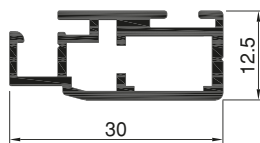
Art.Nr. A1210 Drehrahmenprofil
