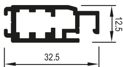
Art.Nr. A1240 Drehrahmenprofil für Duplextür
