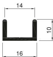
Art.Nr. A1360 U - Profil Führungsschiene für Schiebetüre
