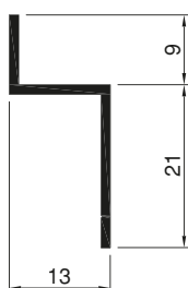
Art.Nr. A7060 Z - Profil Befestigungs-schiene für Spannrahmen
