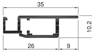
Art.Nr. A1012 Spannrahmenprofil mit Falz 9 mm
