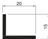
Art.Nr. A8215 L - Winkelprofil 20x15x2
